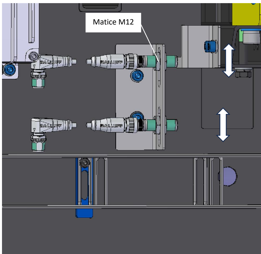
Obr.: Seřízení zdvihu přesuvny
