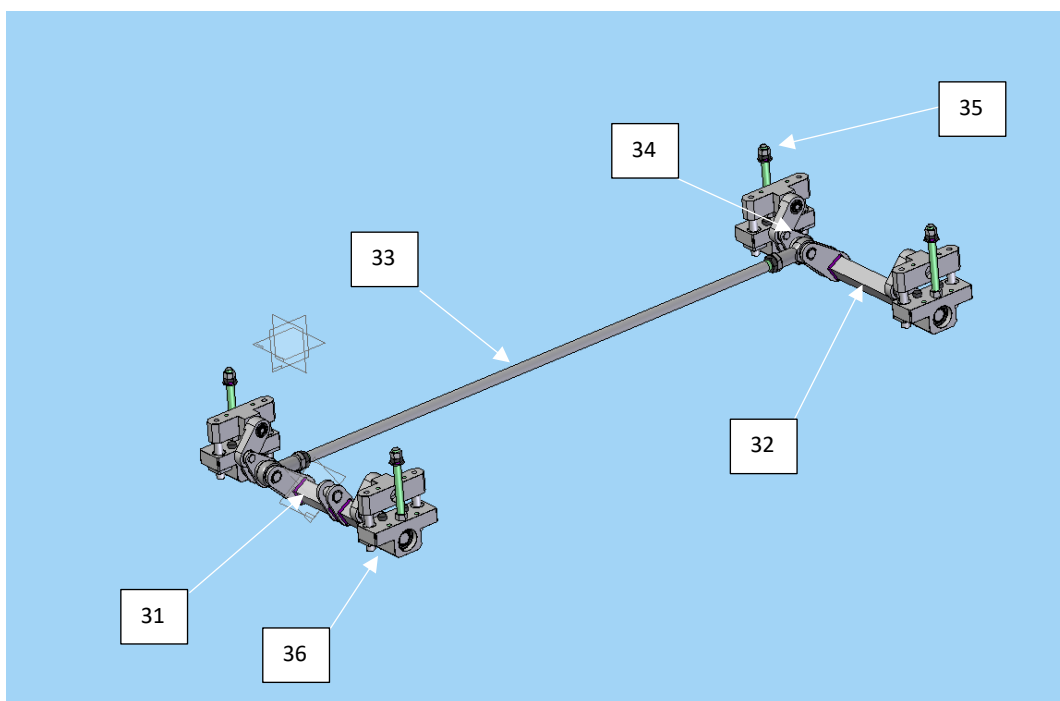
Obr.: Zvedací mechanismu
