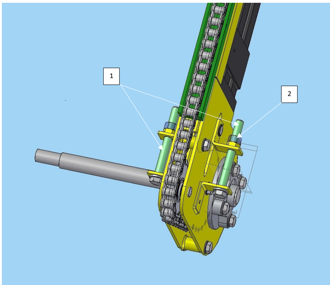
Obr.: Napínání řetězu přesuvny
