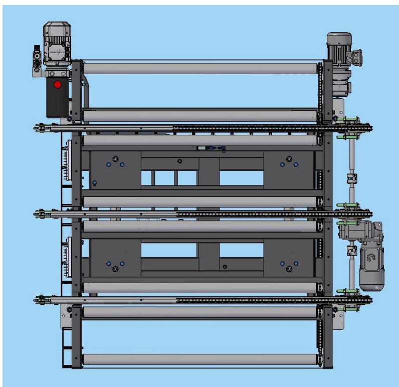
Obr.: Odstrojení stroje dle bodu 3
