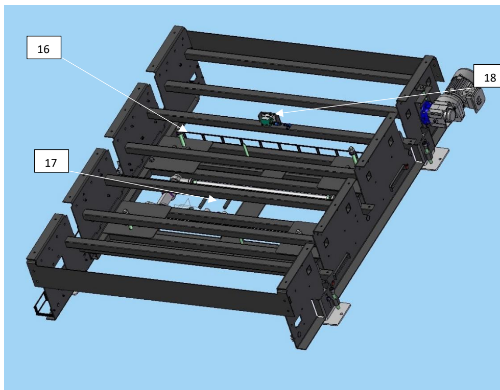
Obr.: Přesuvna – podpěry
