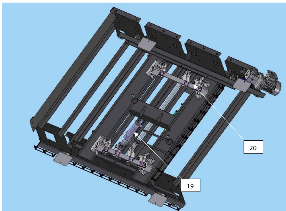
Obr.: Přesuvna, pohled zespodu
