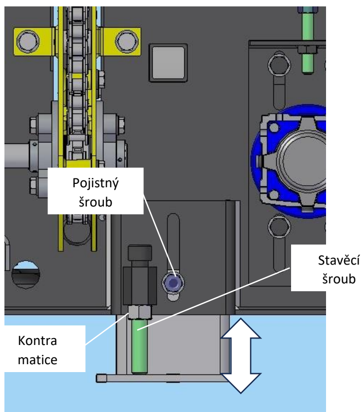
Obr.: Seřízení výšky stroje
