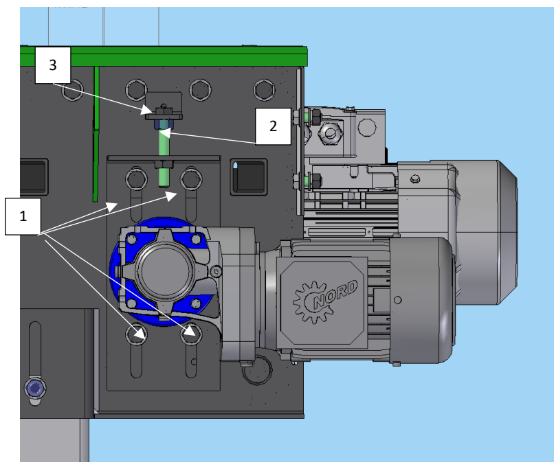
Obr.: Napínání řetězu pohonu válečků
